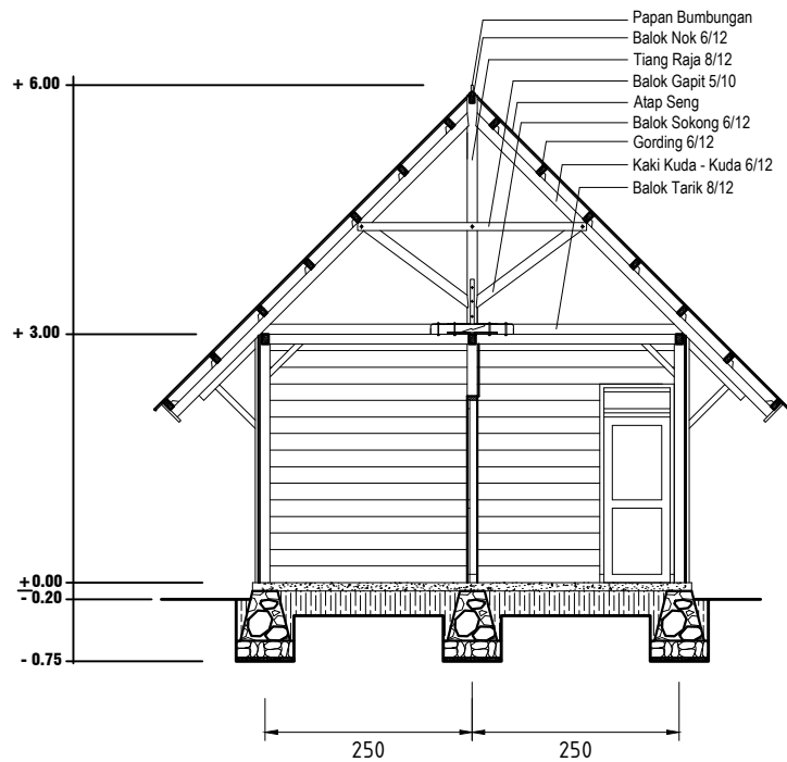
POTONGAN A-A
