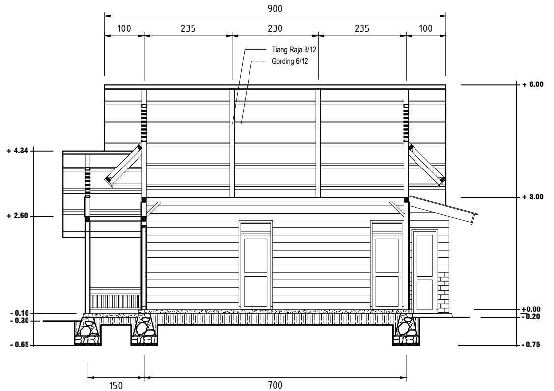
POTONGAN B-B
