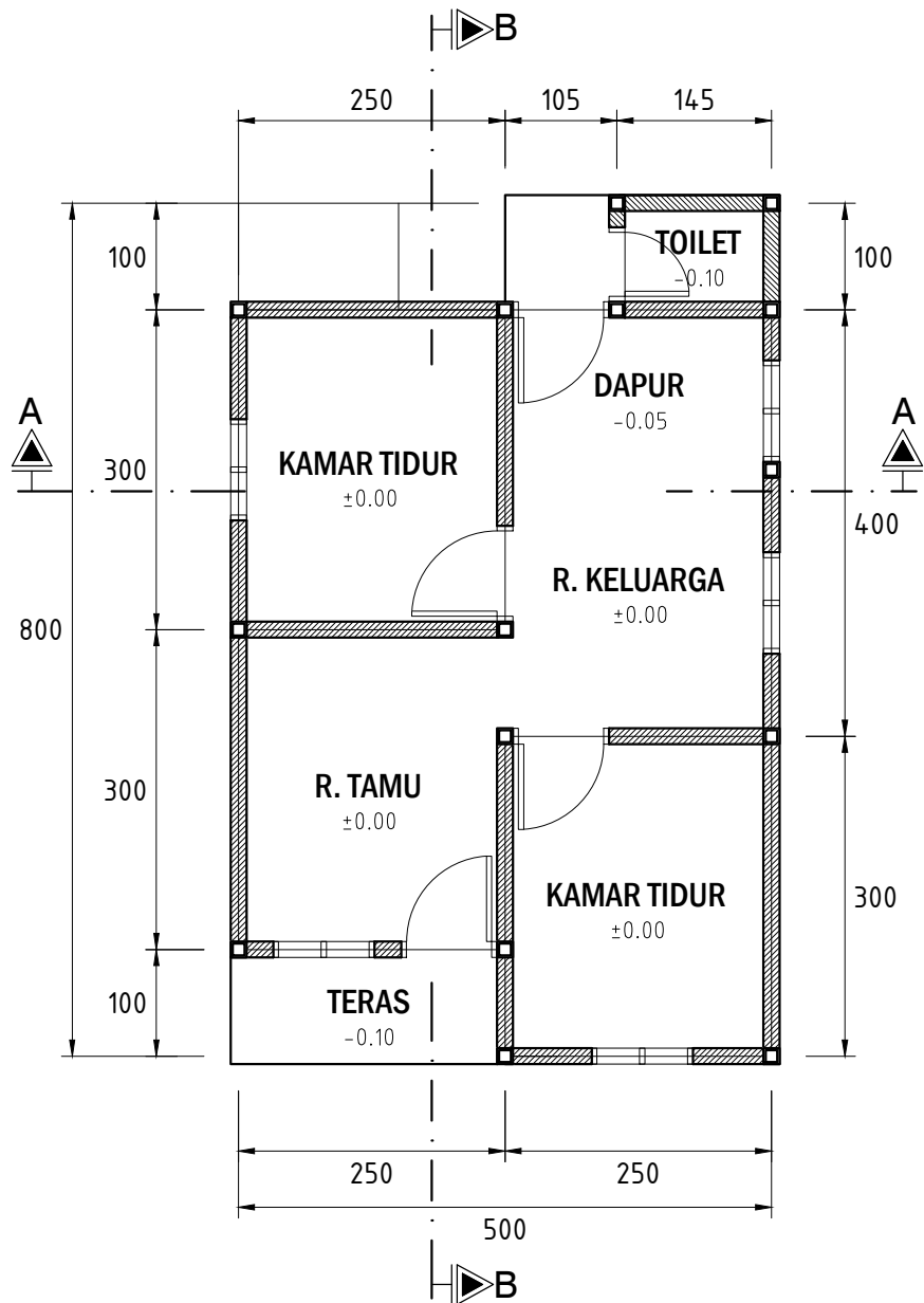
DENAH RUMAH TIPE 36 Skala 1 : 75
